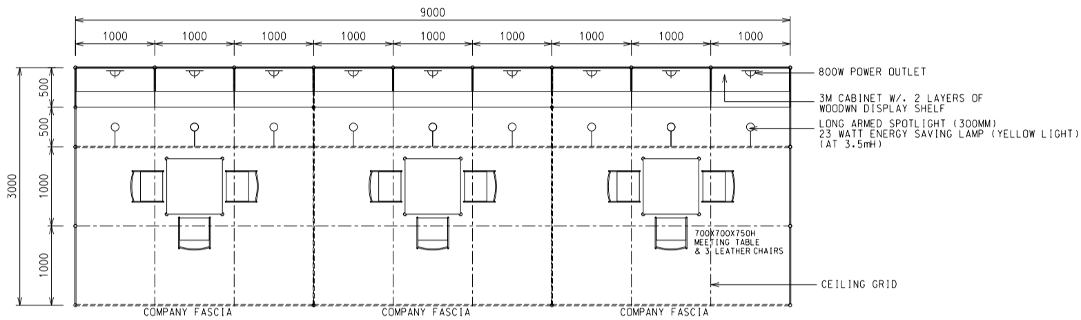
PLAN 9M(W) X 3M(D) X 3.5M(H)
