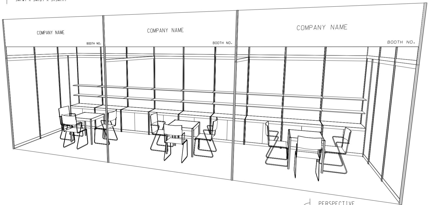
PERSPECTIVE 9M(W) X 3M(D) X 3.5M(H)
